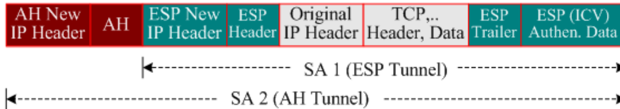
(b) 反覆通道的封包包裝 (IPv4 為範例)
