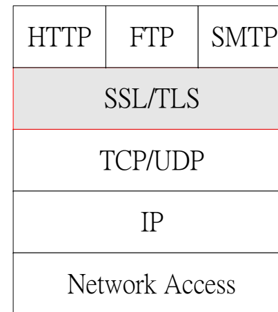
(b) SSL/TLS 協定堆疊
