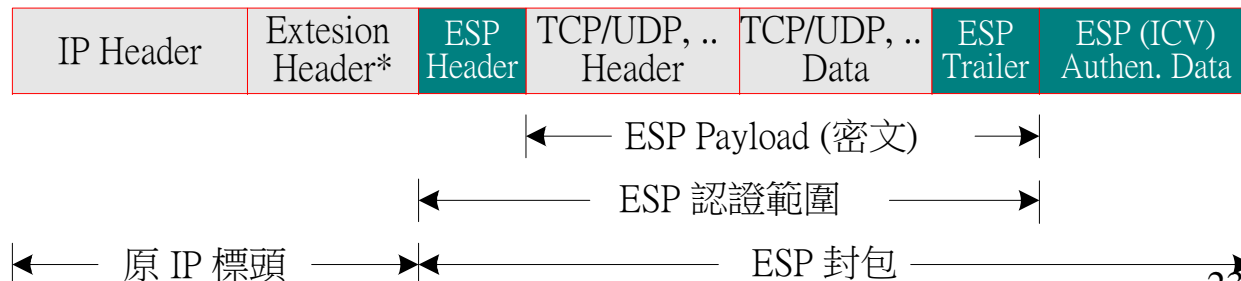
(b) ESP 傳輸模式的 IPSec (IPv6) 封包格式
