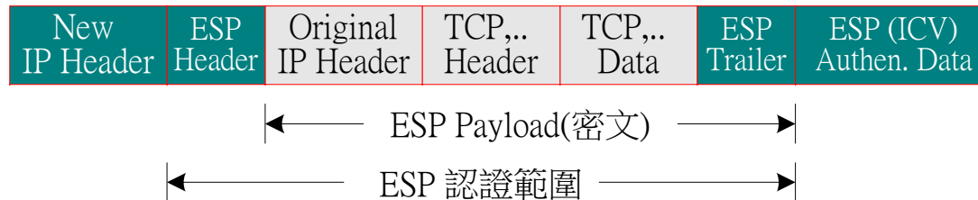
(a) ESP 通道模式的 IPSec (IPv4) 封包格式
