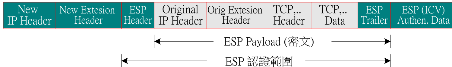
(b) ESP 通道模式的 IPSec (IPv6) 封包格式
