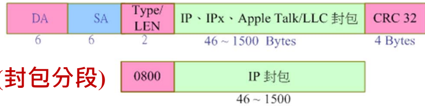
Ethernet II 訊框格式(RFC 890)
