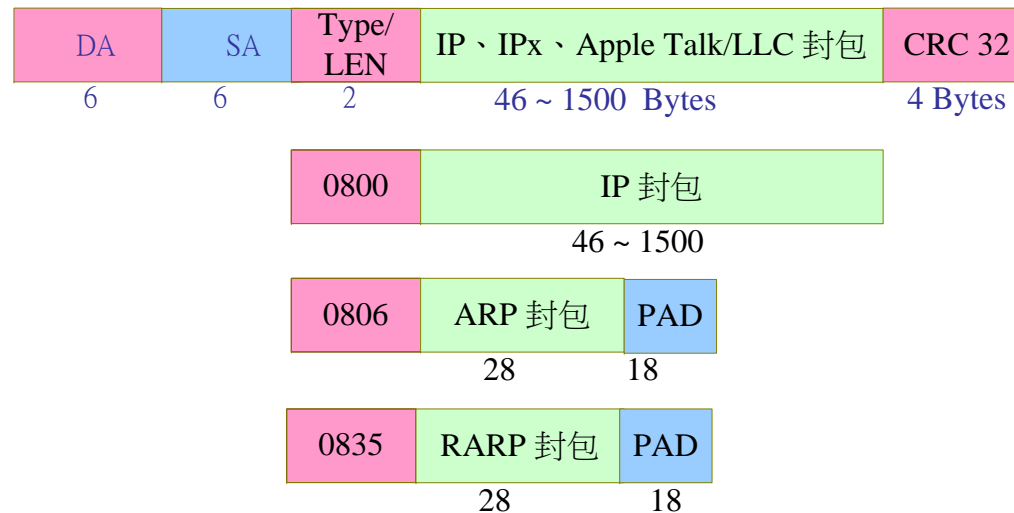
Ethernet II 訊框格式(RFC 890)
