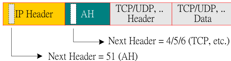
(b) AH 傳輸模式的 IPSec (IPv4) 封包格式
