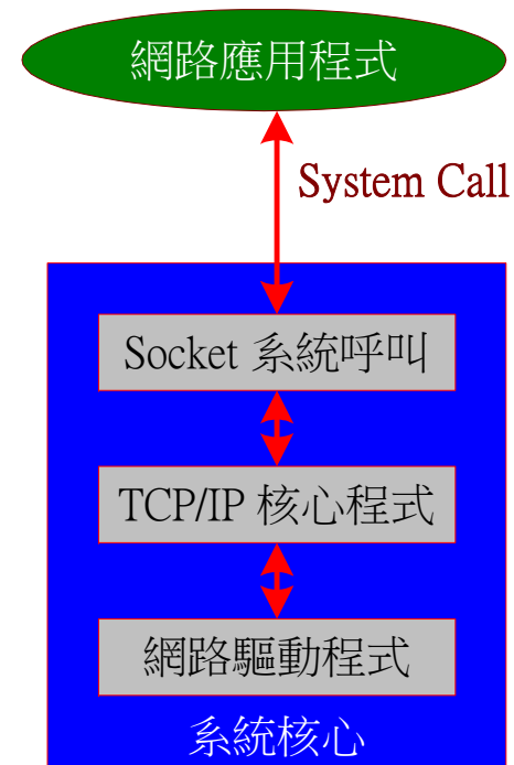
(b) BSD Socket 介面 模組
