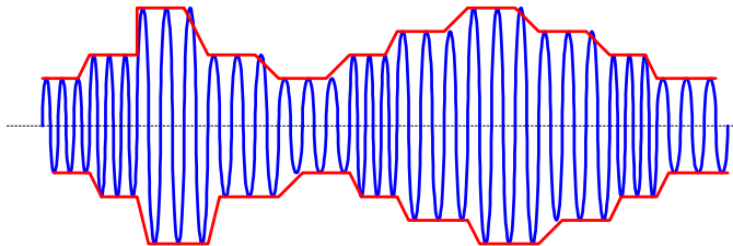
(a) 具有載波之訊號波形
